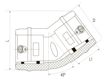
Отводы электросварные ПЭ100 45°
