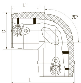
Отводы электросварные ПЭ100 90°
