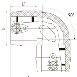
Отводы электросварные ПЭ100 90°
